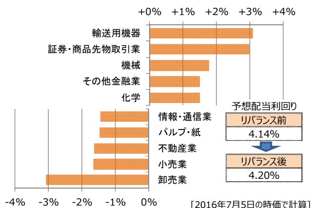
(図表2) 予想配当利回りと業種別構成比の変化
