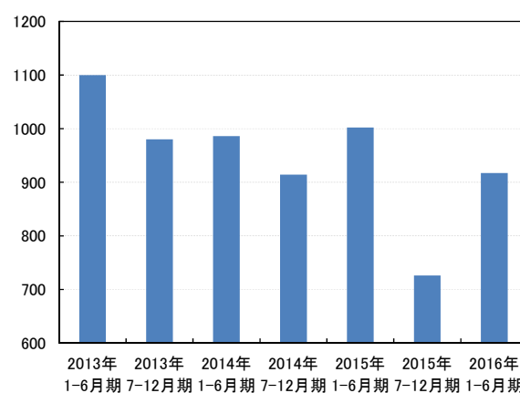
中国の風力発電施設の平均稼働時間 (単位:時間、2013年1-6月期～2016年1-6月期)
